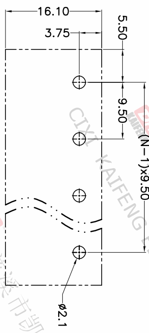
P.C.B.LAYOUT
